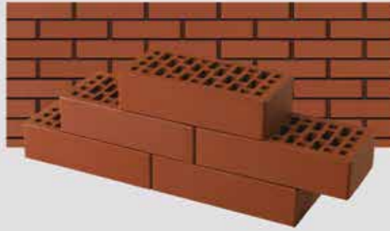
БОРДО 1NF
